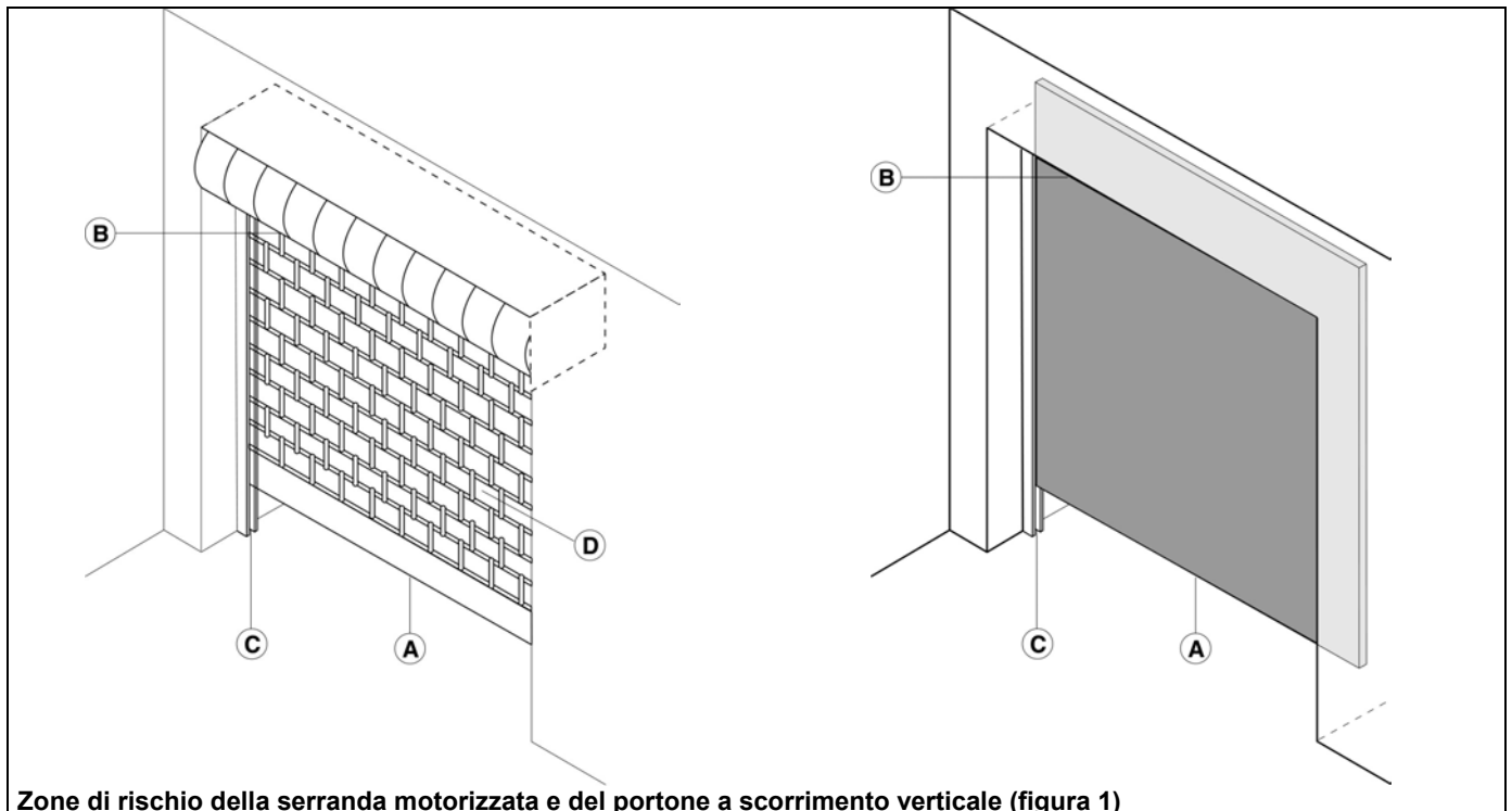
Zone di rischio della serranda motorizzata e del portone a scorrimento verticale (figura 1)
